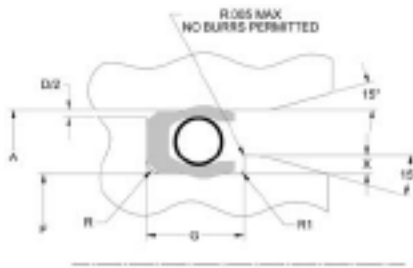
Click Fit Groove — Piston
