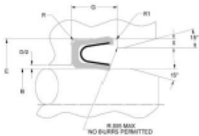
Click Fit Groove — Rod
