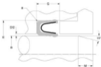
Seal Groove — Rod
